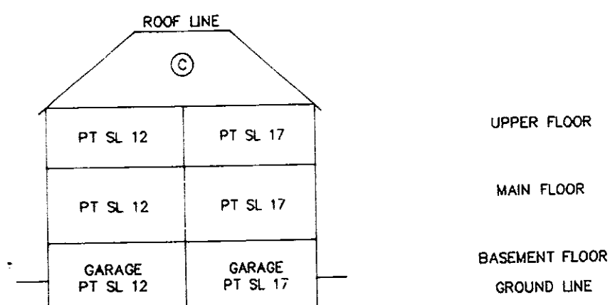
BLOCK 30 : SECTION DD-DD
