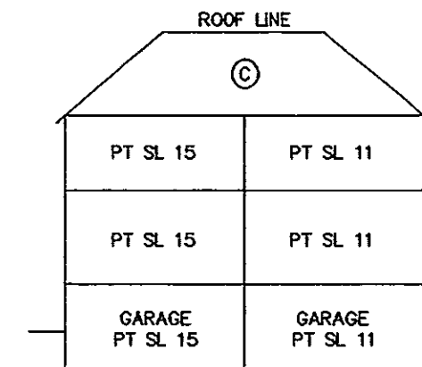
BLOCK 1 : SECTION A-A
