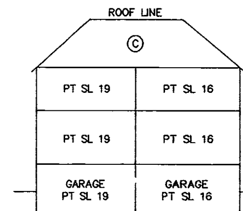
BLOCK 2 : SECTION B-B
